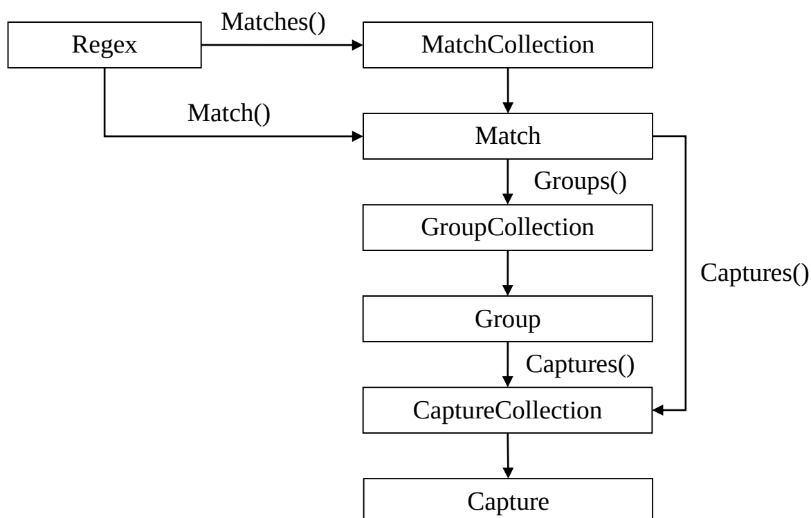
Рис. 2.15 – Схема обработки соответствий при использовании класса Regex
