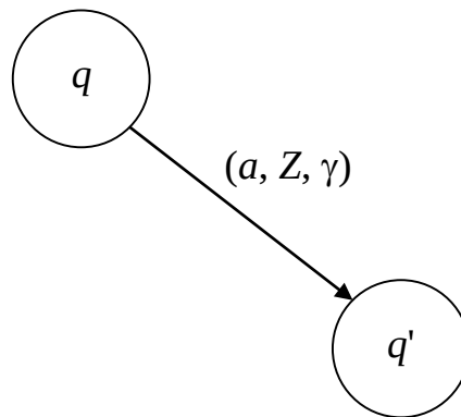
Рис. 2.5 – Переход в графе ДМПА
