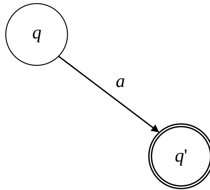
Рис. 2.7 – Переход в конечное состояние ДКА
