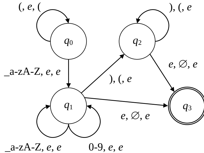
Рис. 2.11 – Граф ДМПА, описывающего идентификатор в скобках
