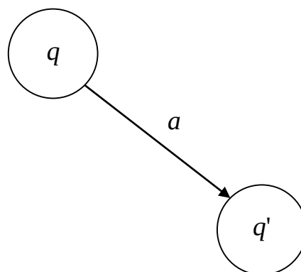
Рис. 2.6 – Переход в графе ДКА
