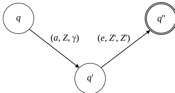
Рис. 2.8 – Переход в конечное состояние ДМПА
