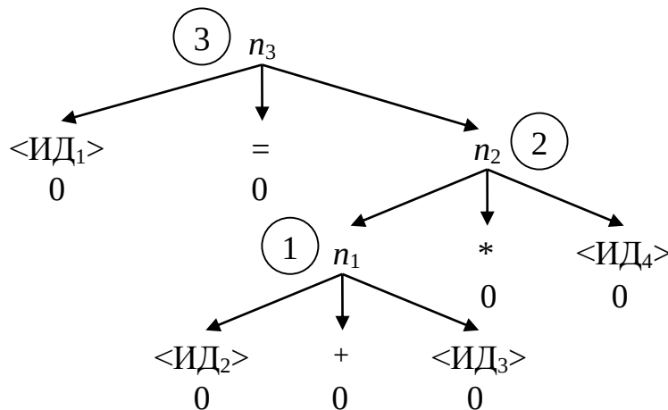
Рис. 2.3 – Дерево с уровнями
