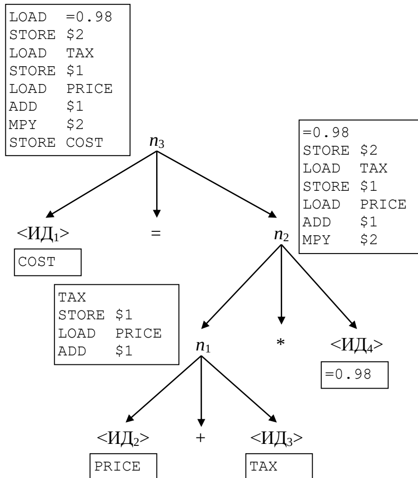
Рис. 2.4 – Дерево с генерированными кодами
