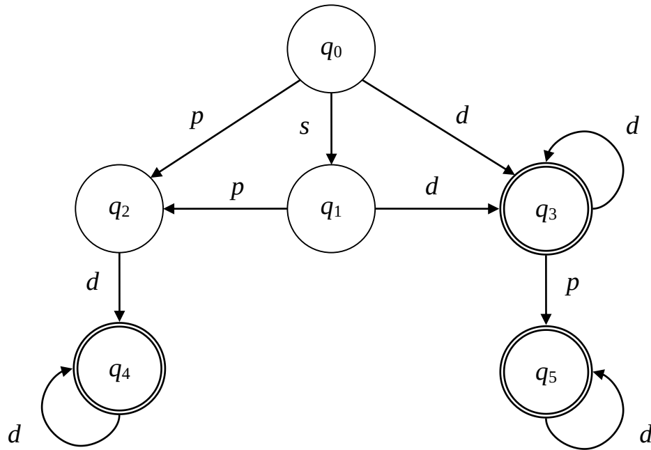
Рис. 2.14 – Граф переходов ДКА, построенный по РВ
