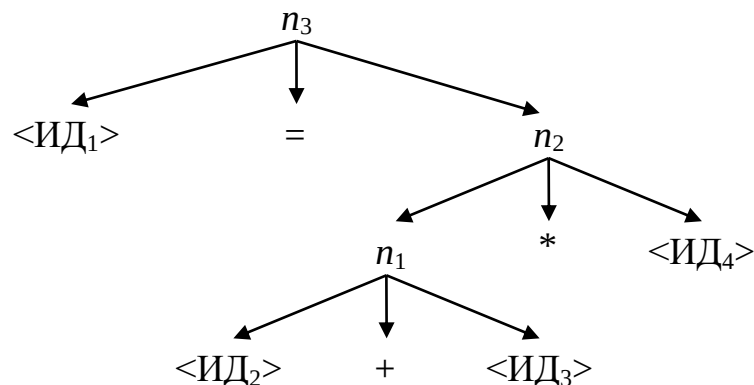
Рис. 2.1 – Последовательность действий при вычислении выражения
