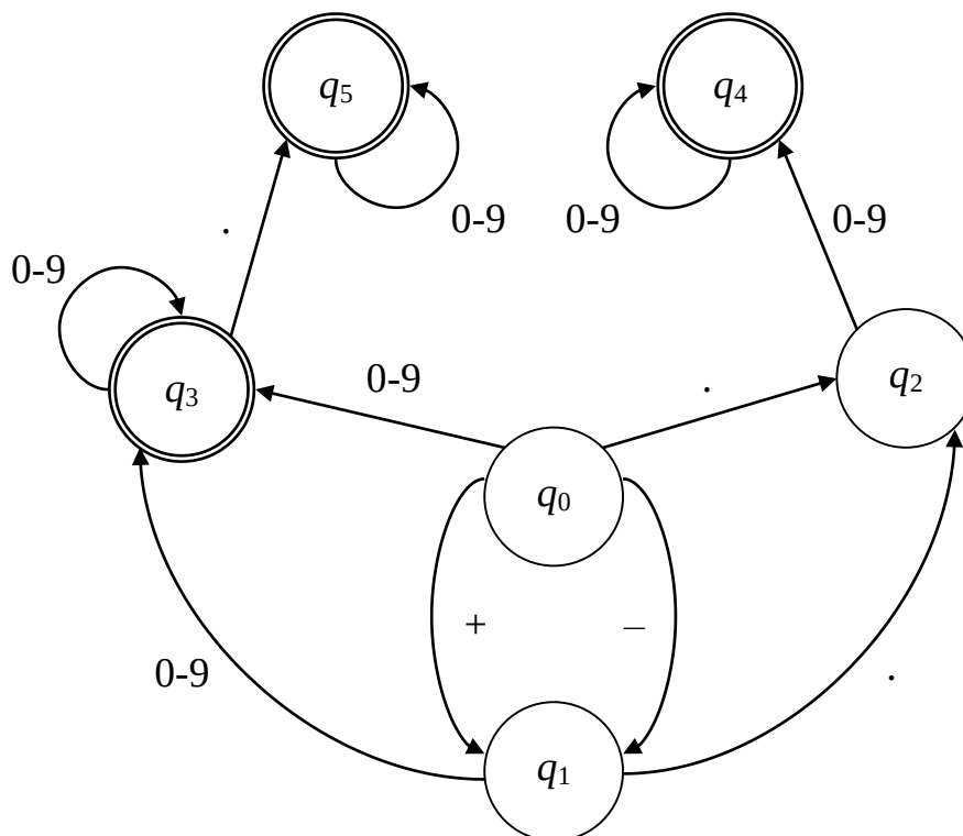
Рис. 2.9 – Граф ДКА, описывающего число с фиксированной точкой
