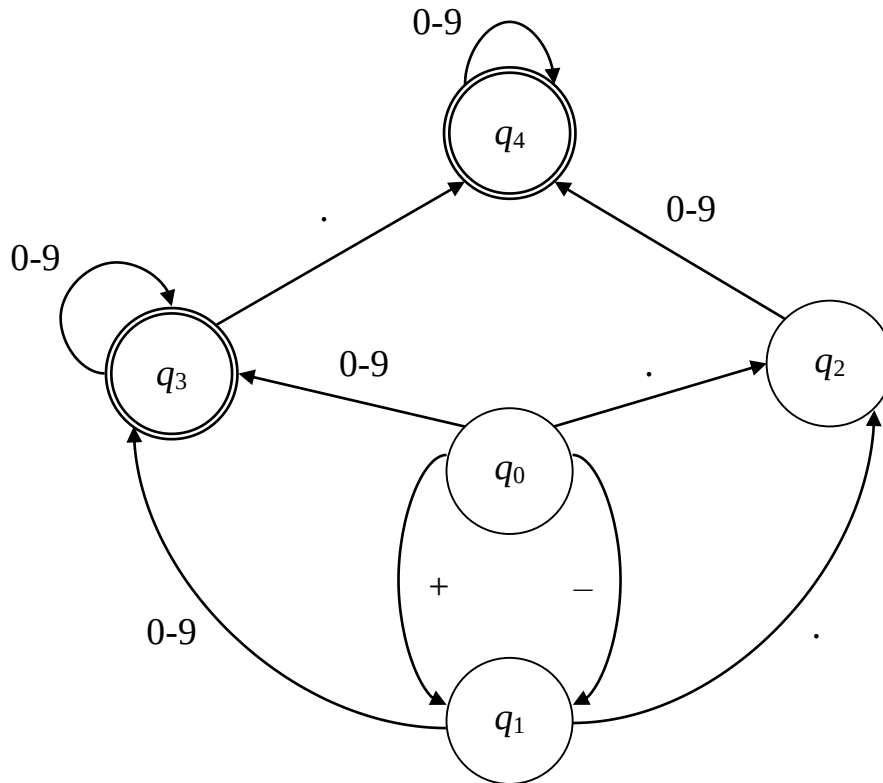
Рис. 2.10 – Минимизированный граф ДКА, описывающего число с фиксированной точкой
