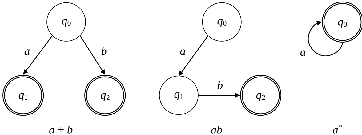
Рис. 2.12 – Сопоставление графа переходов ДКА и базовых операций РВ
