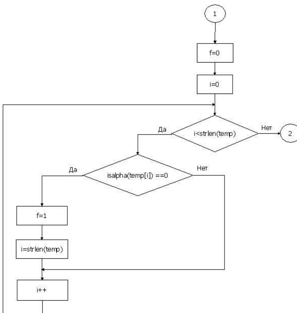
Рис. 5.1 – Алгоритм проверки символов
