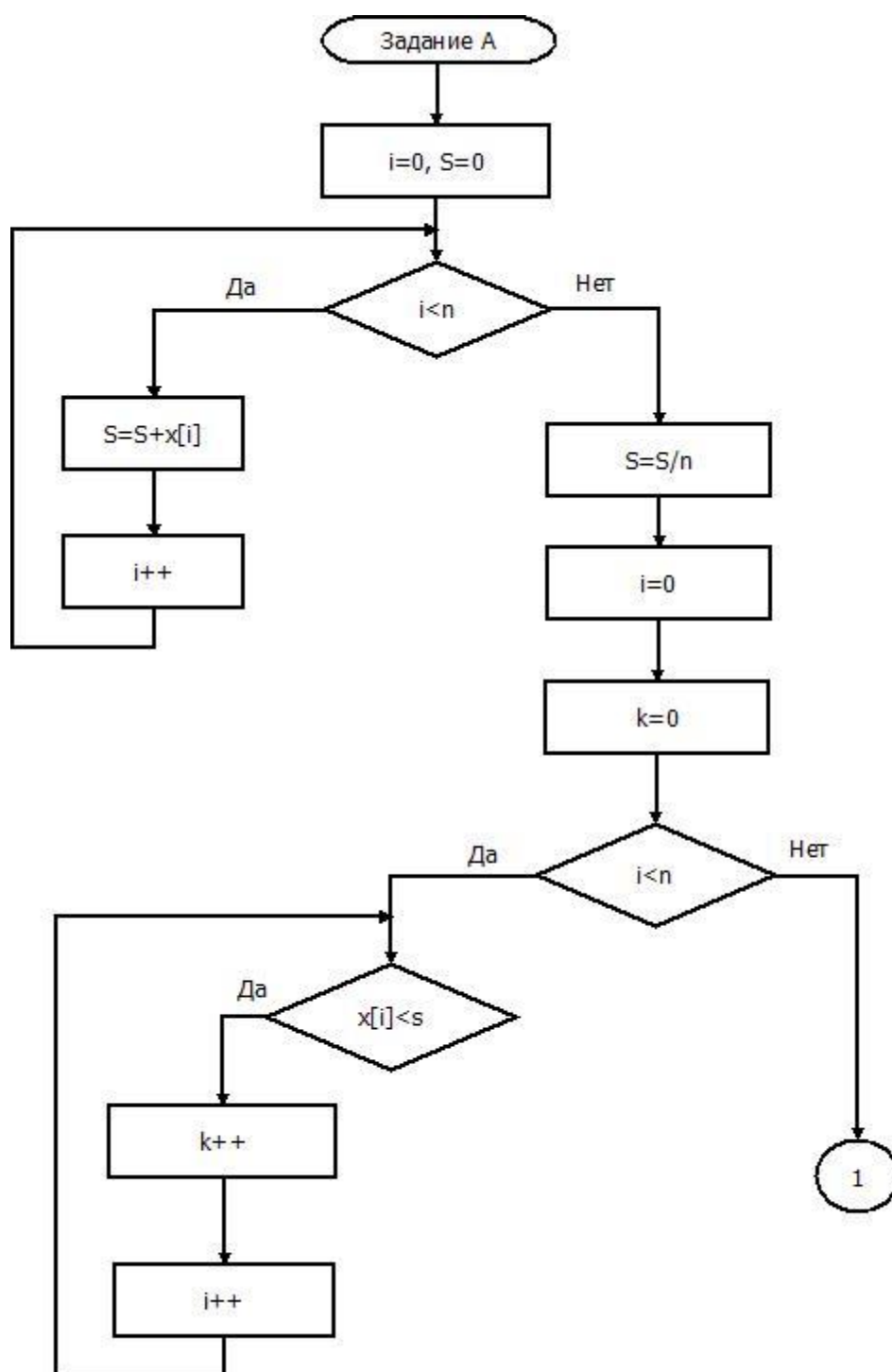
Рис. 3.2 – Алгоритм задания А
