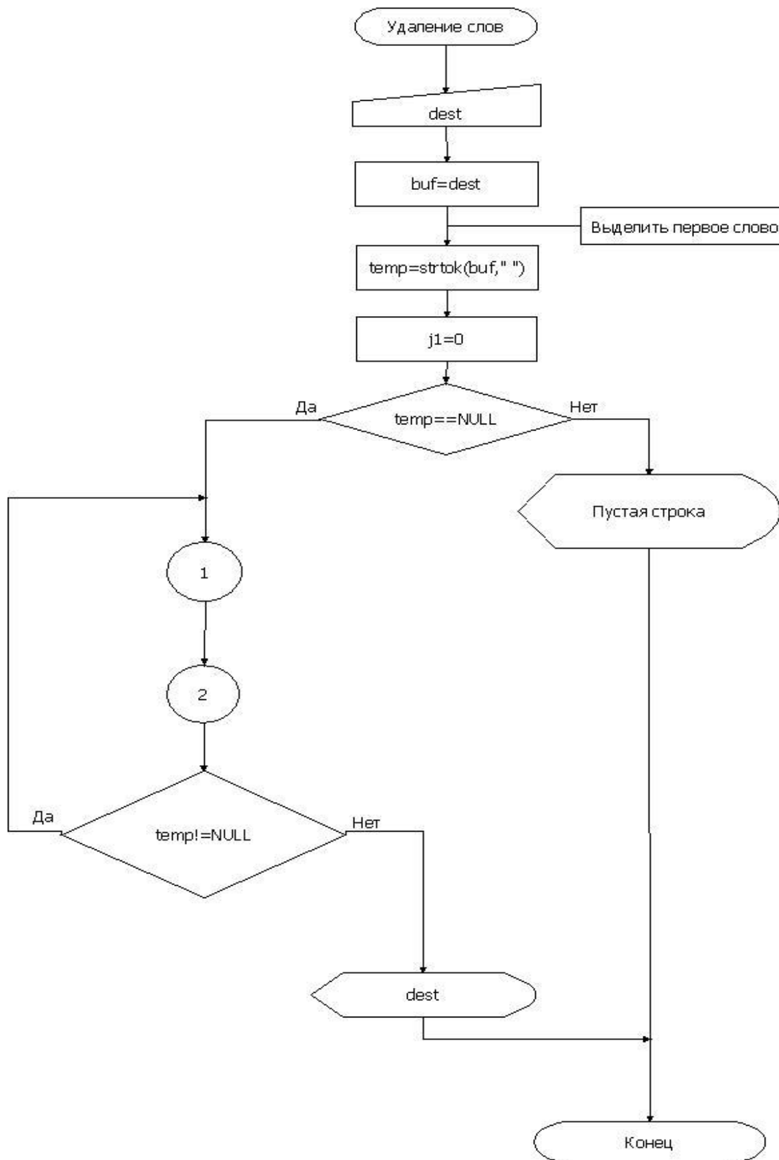
Рис. 5.3 – Алгоритм удаления слов
