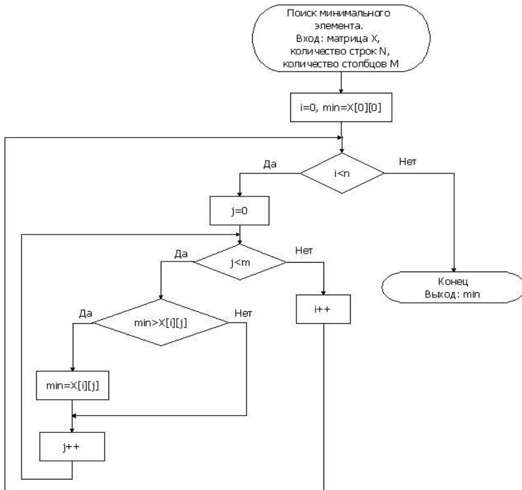
Рис. 4.3 – Поиск минимального элемента
