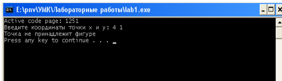
Рис. 1 – Результаты тестирования
