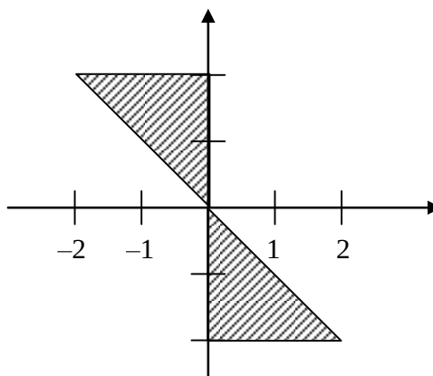
Рис. 2.3 – Пример 1
