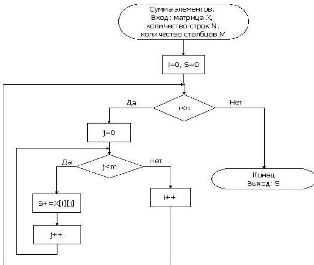
Рис. 4.1 – Поиск суммы элементов матрицы
