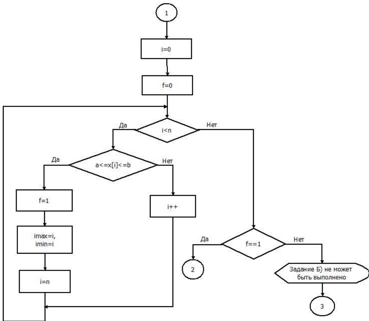
Рис. 3.3 – Нахождение первого встреченного элемента массива x \in [a, b]
