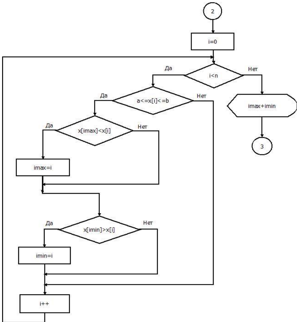
Рис. 3.4 – Поиск минимального и максимального значения
