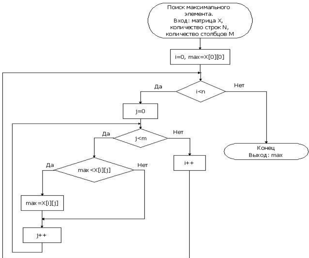
Рис. 4.2 – Поиск максимального элемента матрицы
