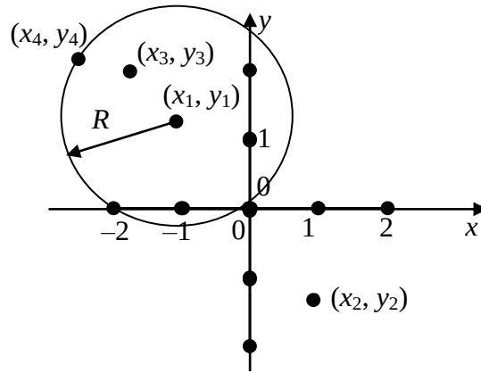
Рис. 2.2 – Расположение точки относительно окружности R^2 = (x - x_1)^2 + (y - y_1)^2
