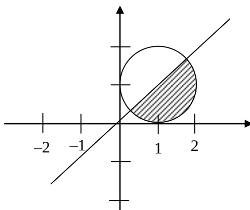
Рис. 2.4 – Пример 2
