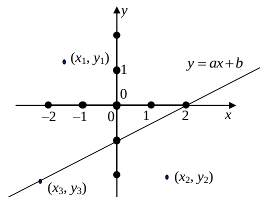
Рис. 2.1 – Расположение точки относительно прямой y = ax + b
