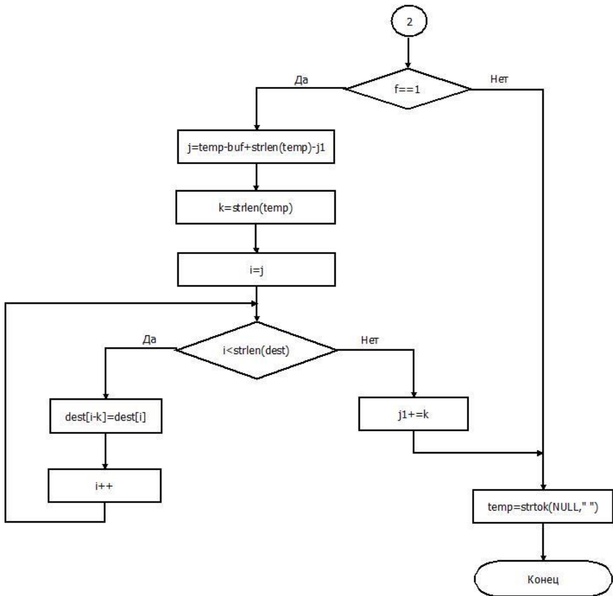
Рис. 5.2 – Алгоритм перемещения символов в начало строки
