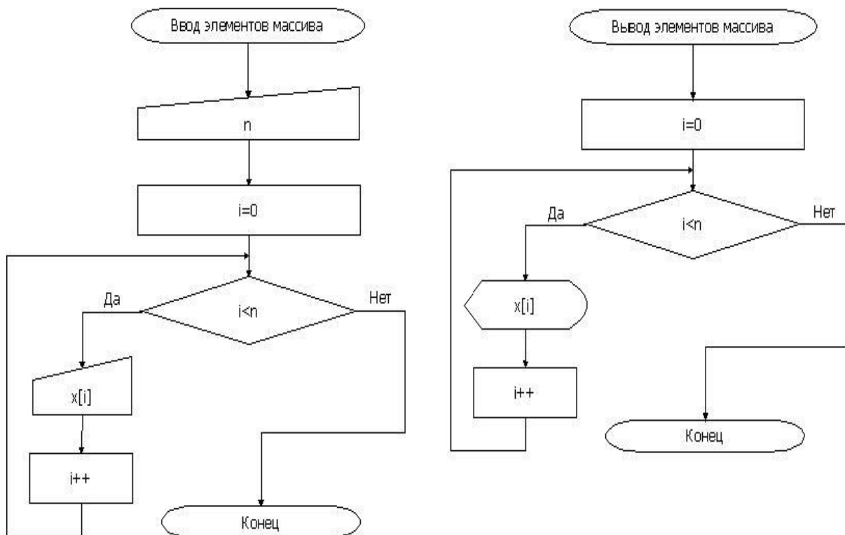
Рис. 3.1 – Ввод и вывод элементов массива
