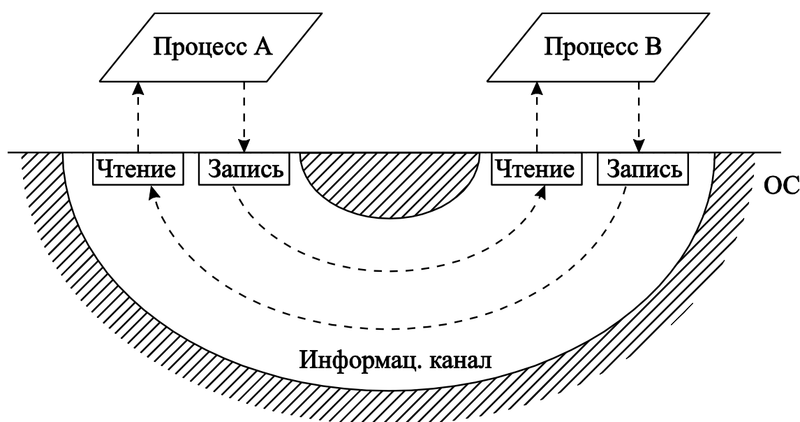
Рис. 3.6 – Взаимодействие процессов через информационный канал
