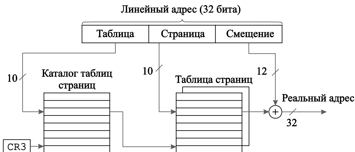
Рис. 6.10 – Преобразование линейного виртуального адреса в реальный
