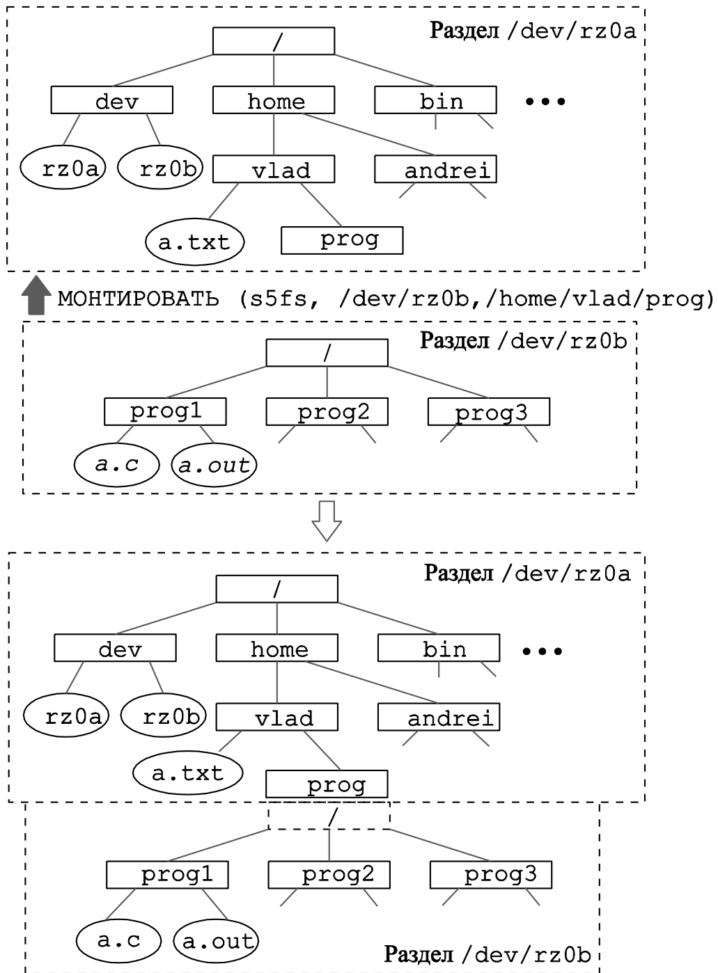
Рис. 7.4 – Пример монтирования реальной файловой системы
