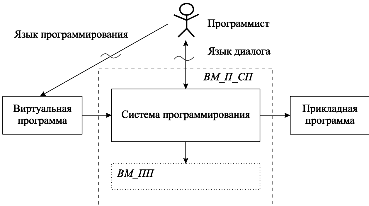
Рис. 2.9 – Виртуальная машина пользователя системы программирования: ВМ_П_СП – виртуальная машина пользователя системы программирования; ВМ_ПП – виртуальная машина прикладной программы
