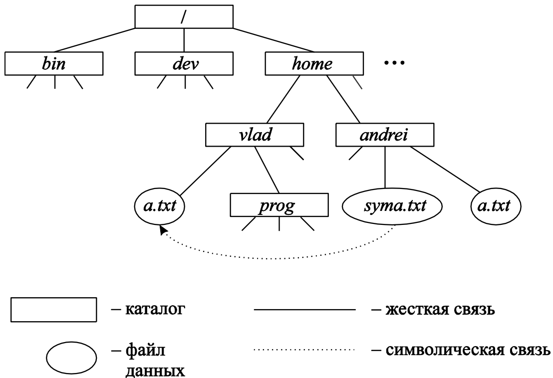
Рис. 2.7 – Фрагмент файловой структуры UNIX
