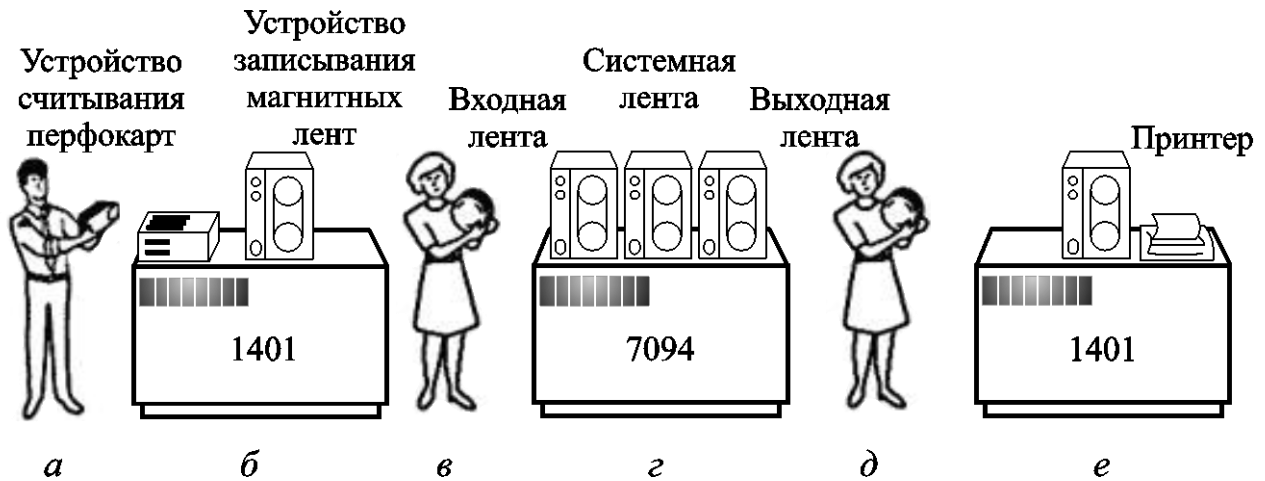
Рис. 1.1 – Ранняя система пакетной обработки: программист приносит карты для IBM 1401 ( a ); IBM 1401 записывает пакет заданий на магнитную ленту ( б ); оператор переносит входные данные на ленте к IBM 7094 ( в ); IBM 7094 выполняет вычисления ( г ); оператор переносит ленту с выходными данными на IBM 1401 ( д ); IBM 1401 печатает выходные данные ( e )
