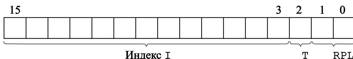
Рис. 6.4 – Структура сегментного регистра в защищенном режиме.
