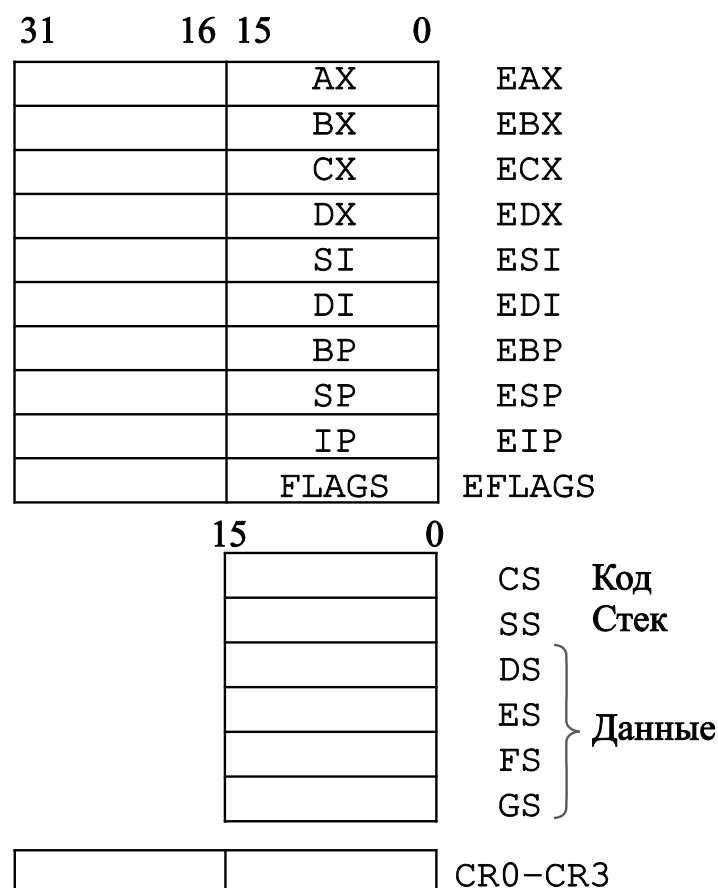
Рис. 6.2 – Регистры процессора i80386
