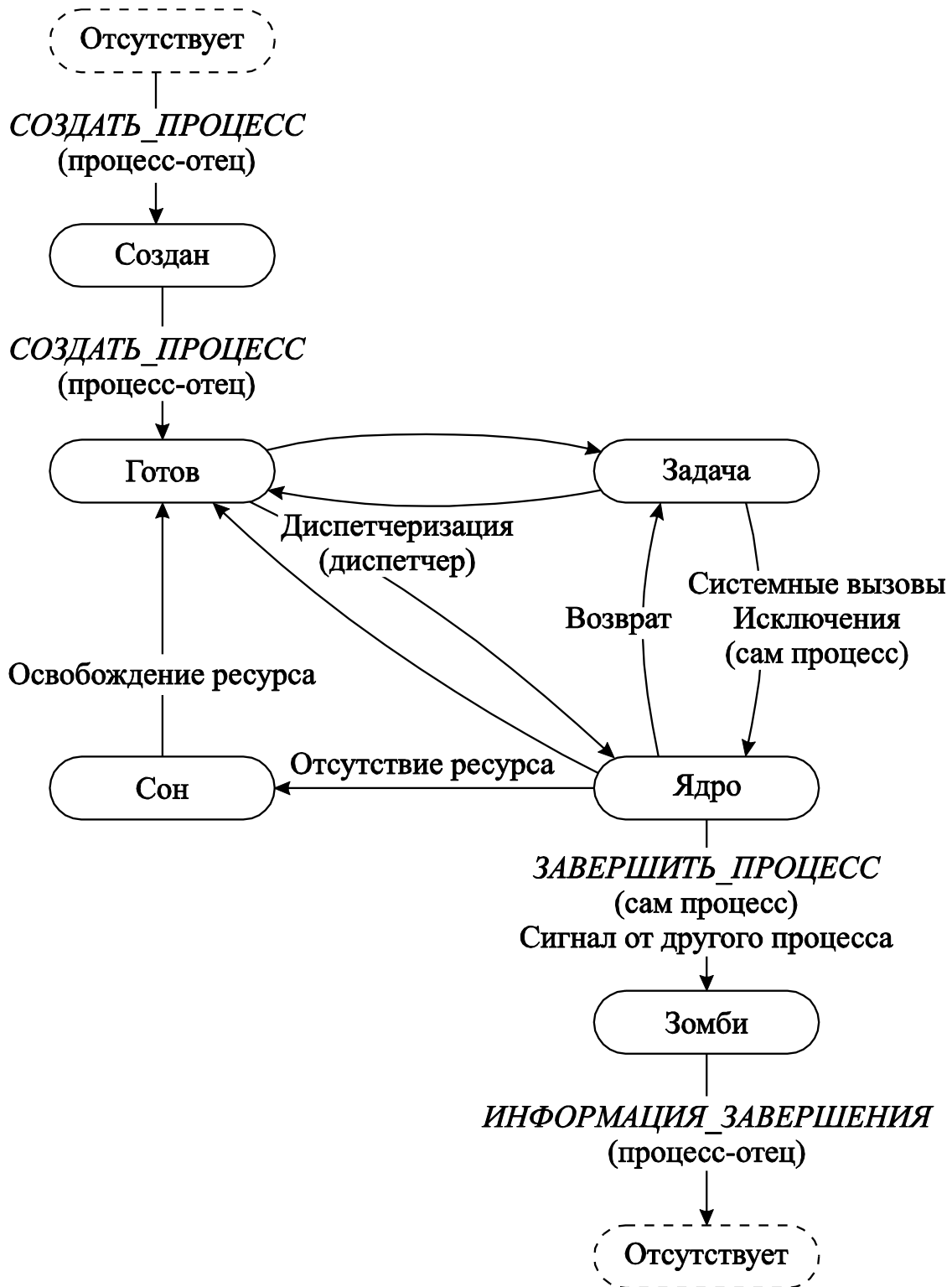
Рис. 5.1 – Состояния процесса
