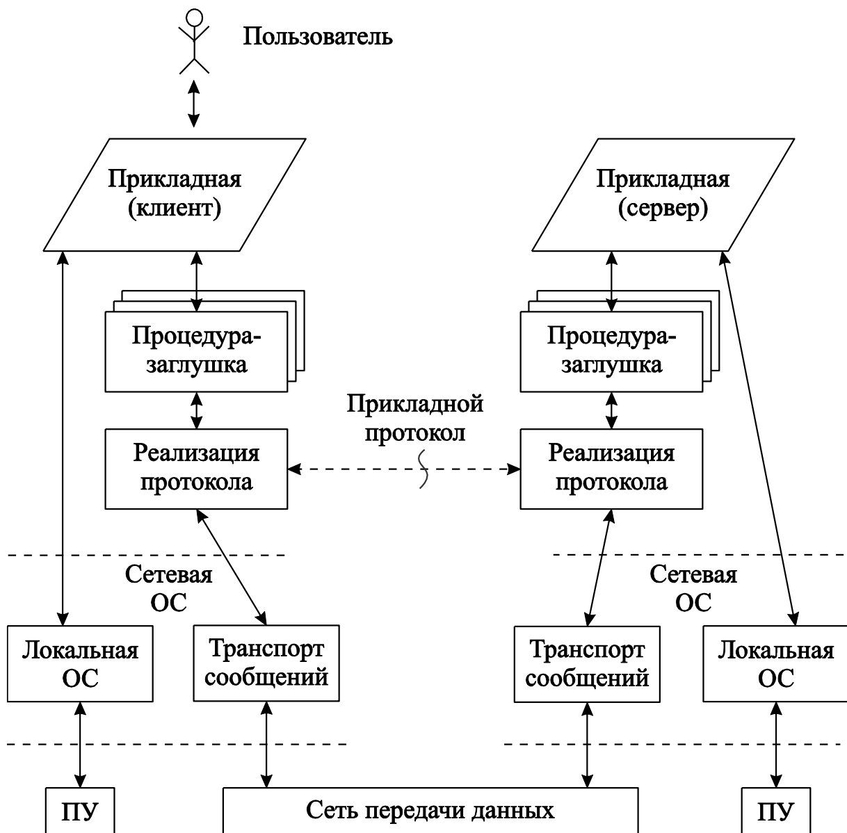
Рис. 4.5 – Распределенная программа с удаленным вызовом процедур
