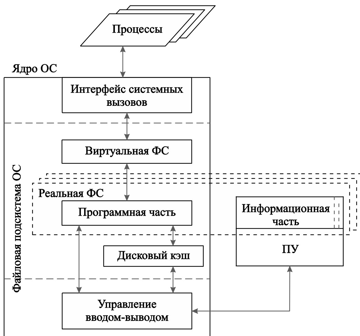
Рис. 7.1 – Структура файловой подсистемы ОС
