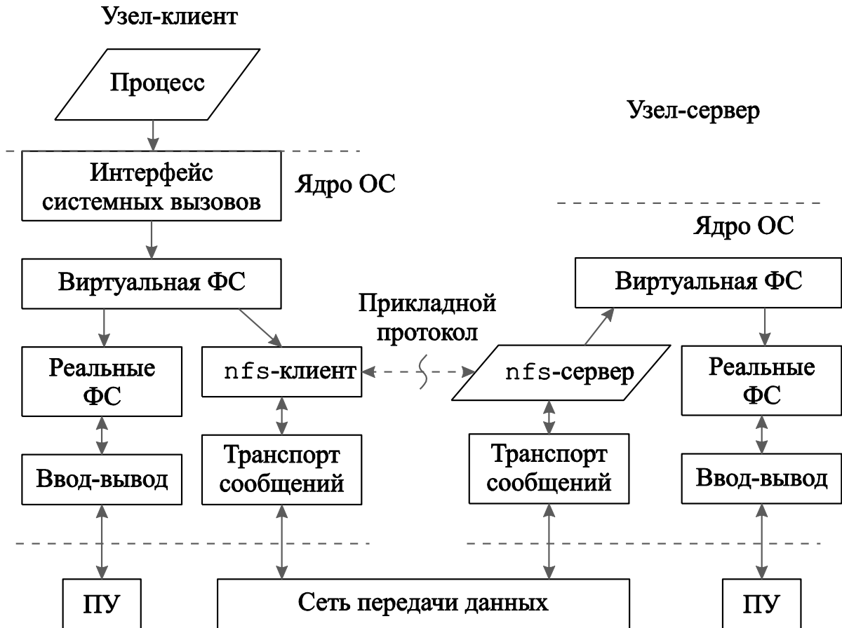
Рис. 7.5 – Распределенная реальная файловая система nfs
