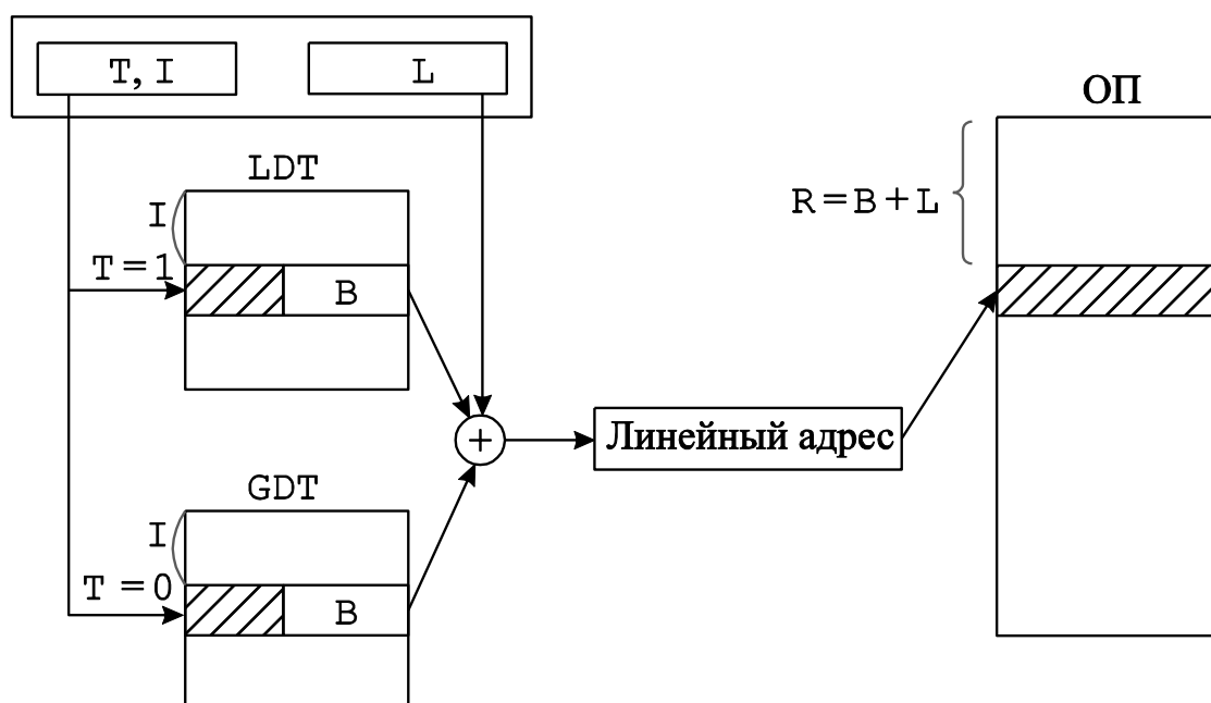
Рис. 6.3 – Преобразование виртуального сегментного адреса в реальный при отсутствии аппаратуры управления страницами.
