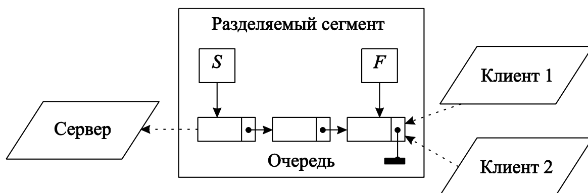
Рис. 3.3 – Три процесса разделяют сегмент памяти
