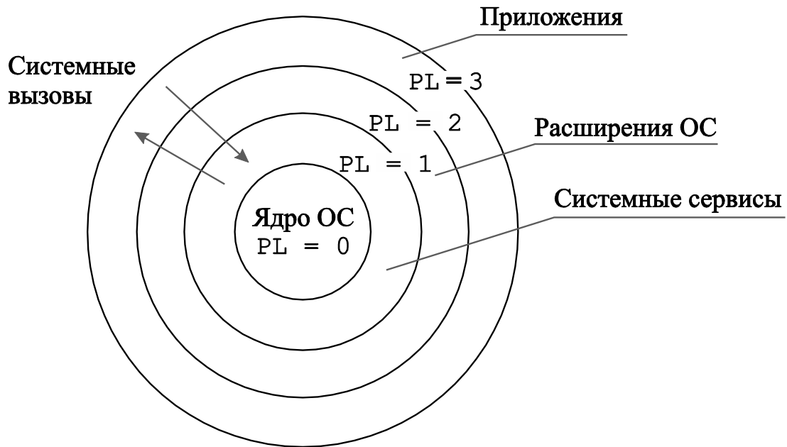
Рис. 6.9 – Возможное распределение программ ОС по кольцам защиты
