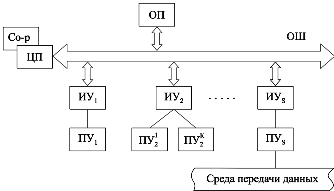
Рис. 2.1 – Однопроцессорная ЭВМ с общей шиной
