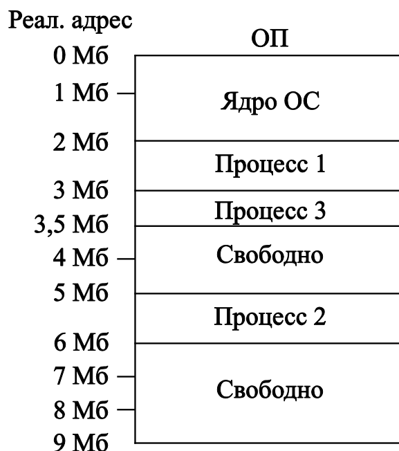
Рис. 6.8 – Пример распределения памяти
