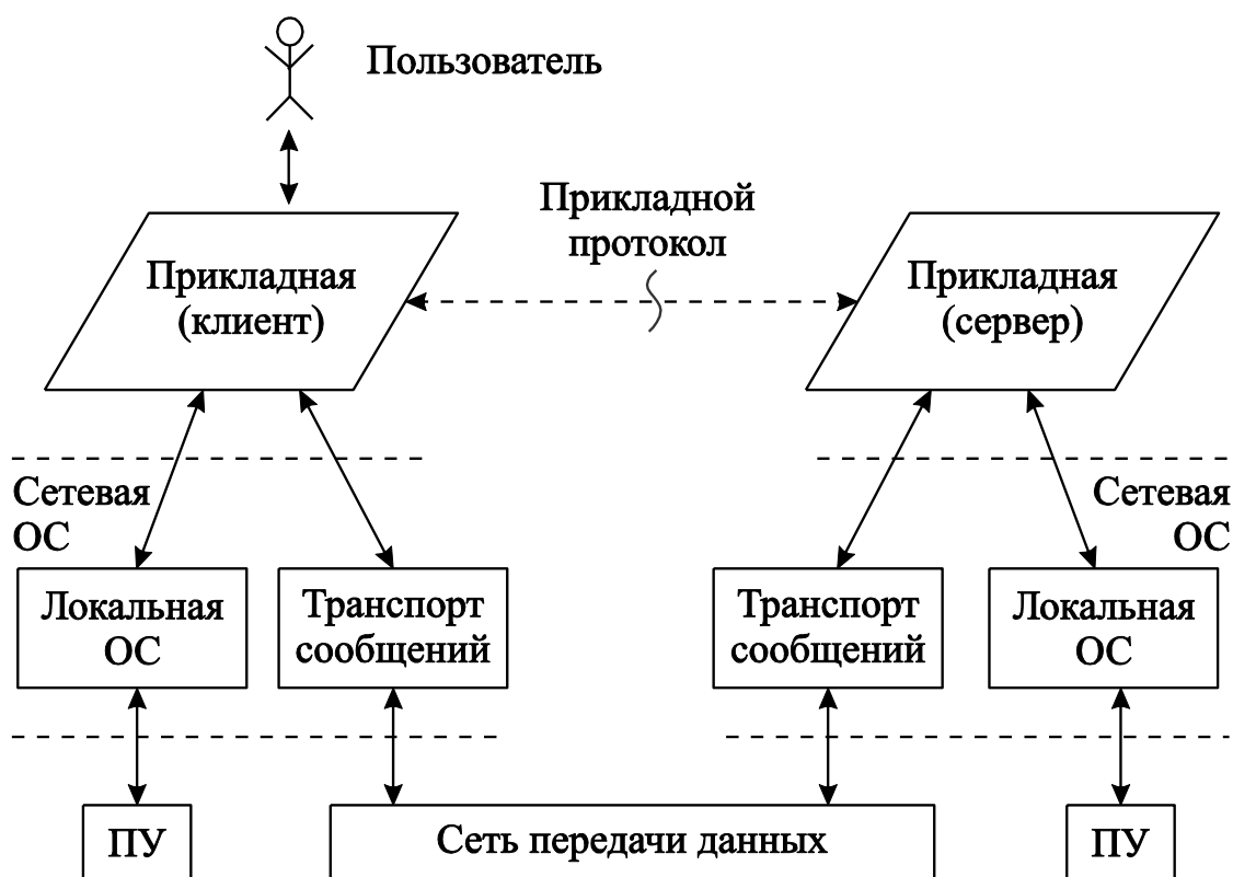
Рис. 4.4 – Выполнение распределенной программы в сети
