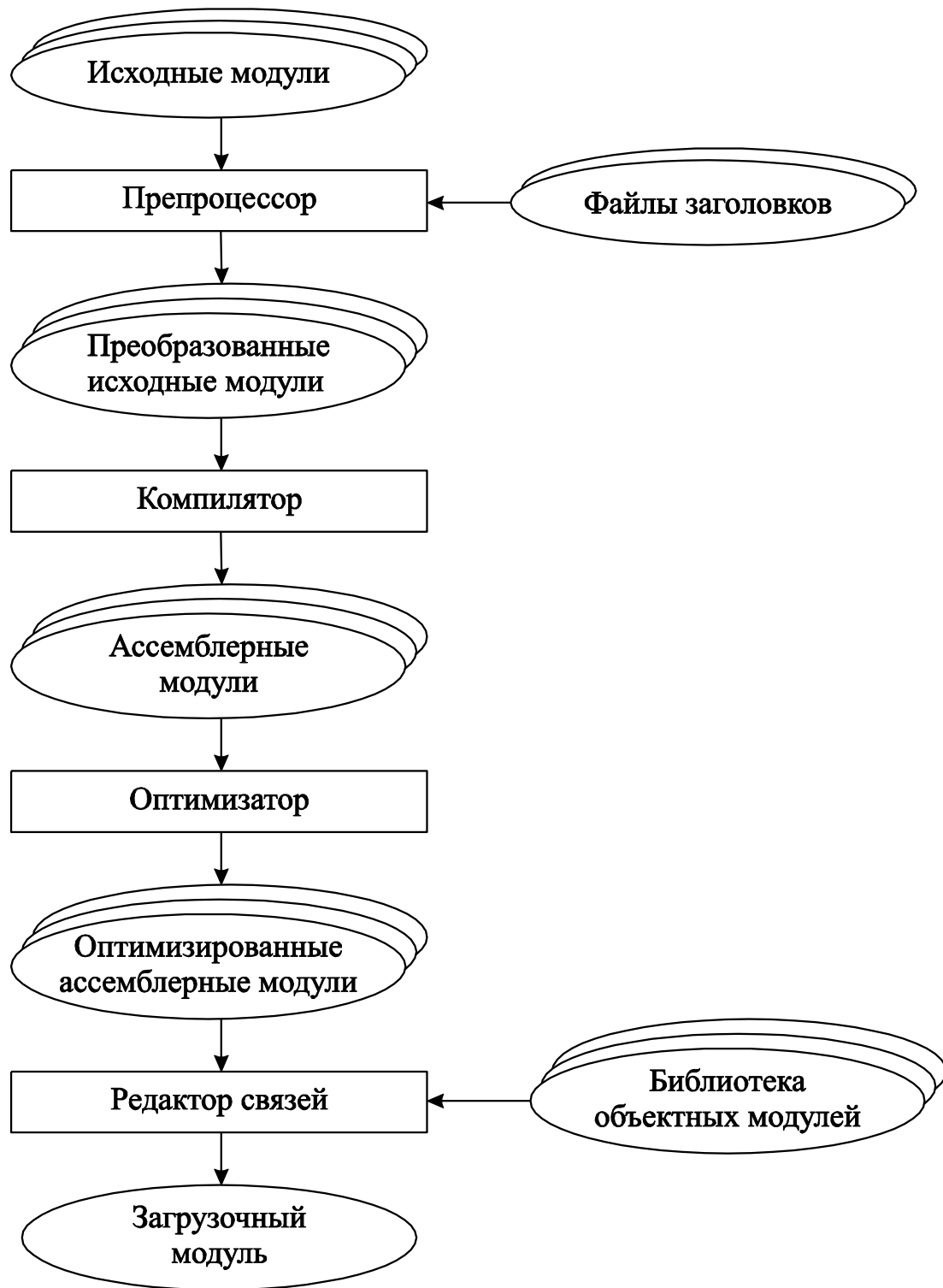
Рис. 2.8 – Преобразование исходной программы в загрузочный модуль
