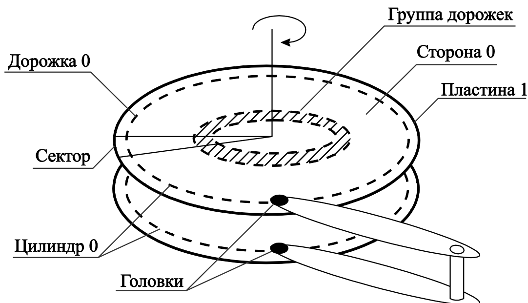
Рис. 7.3 – Упрощенное представление магнитного диска
