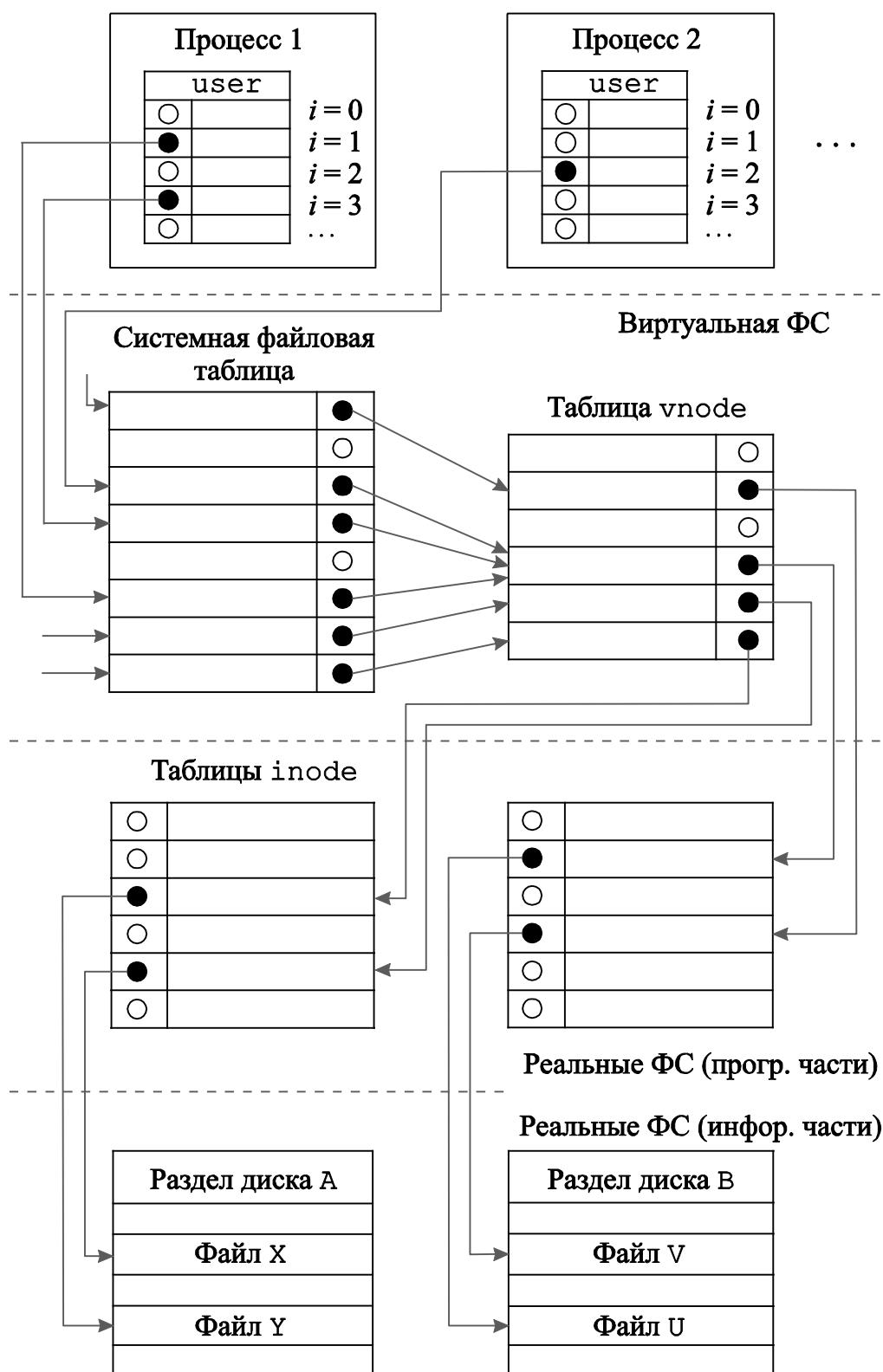
Рис. 7.2 – Системные структуры данных для доступа процессов к файлам
