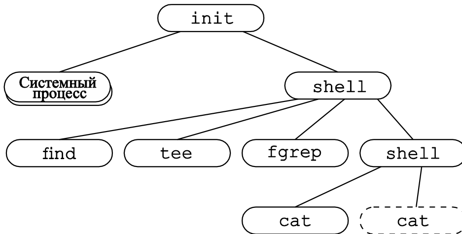
Рис. 3.1 – Пример дерева процессов
