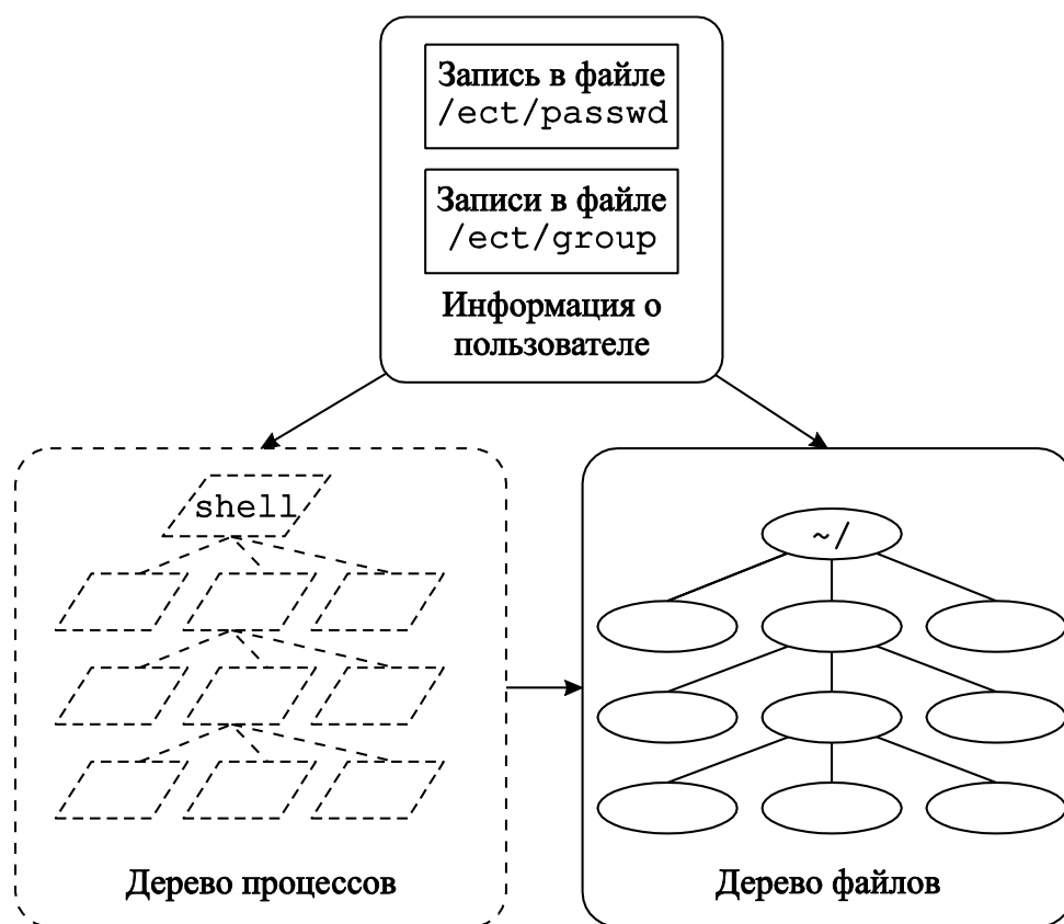
Рис. 4.2 – Информационный след пользователя в системе
