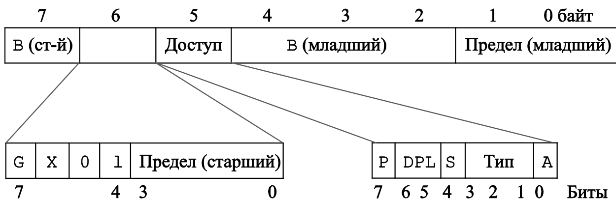
Рис. 6.5 – Структура дескриптора сегмента
