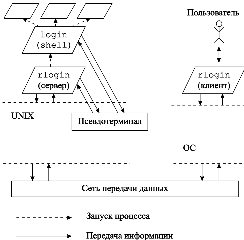
Рис. 4.1 – Доступ удаленного пользователя в UNIX-систему
