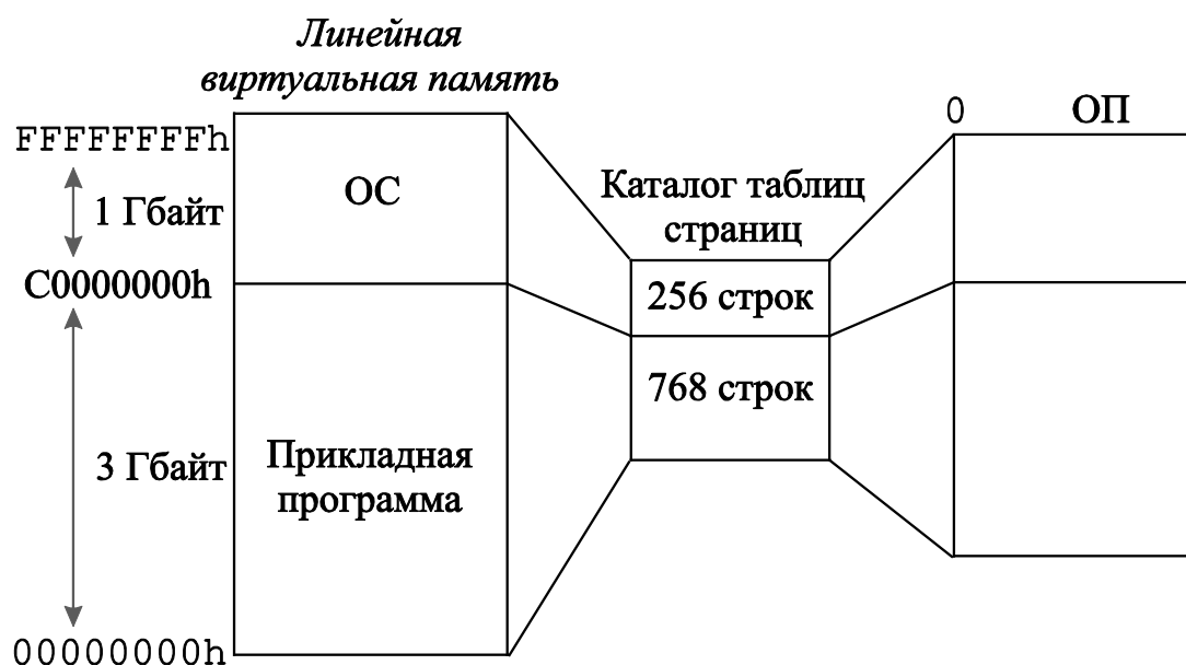
Рис. 6.12 – Отображение линейной виртуальной памяти на реальную ОП
