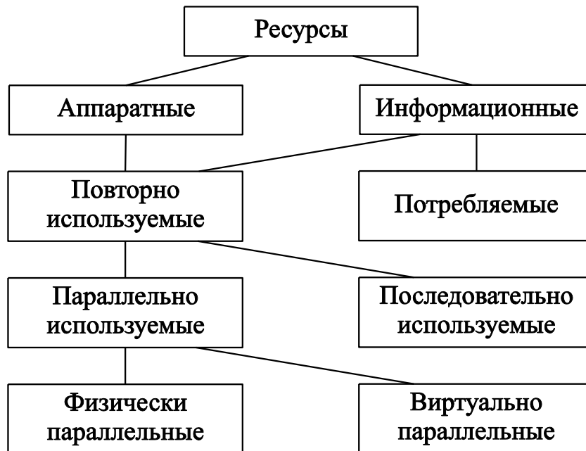
Рис. 3.2 – Классификация ресурсов
