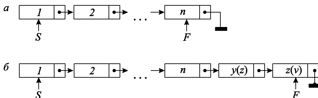
Рис. 3.4 – Состояния очереди:
