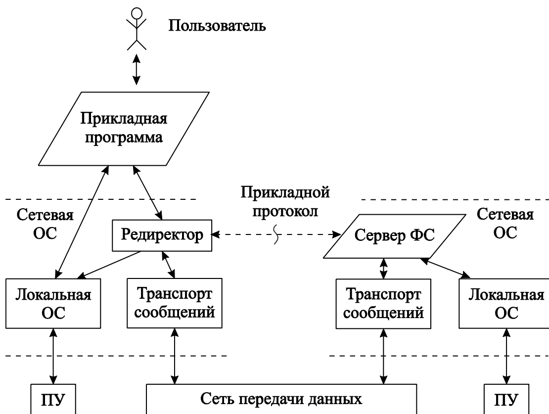
Рис. 4.6 – Сетевое обслуживание локальной прикладной программы
