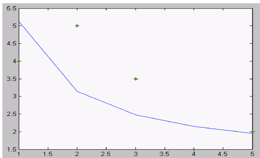
Рис.11.2. Исходные данные и график для гиперболической функции
