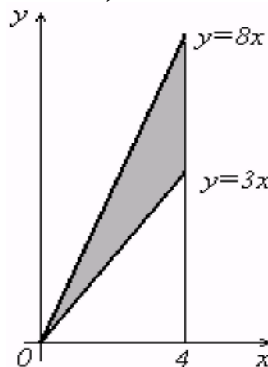
Рис. 10.1. Область D = \{ x=0, x=4, y=3x, y=8x \}
