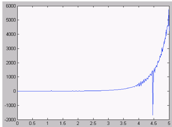
Рис. 16.2. Численное решение интегрального уравнения Вольтерра
