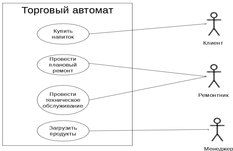
Рис. 4.19 – Варианты использования для торгового автомата
