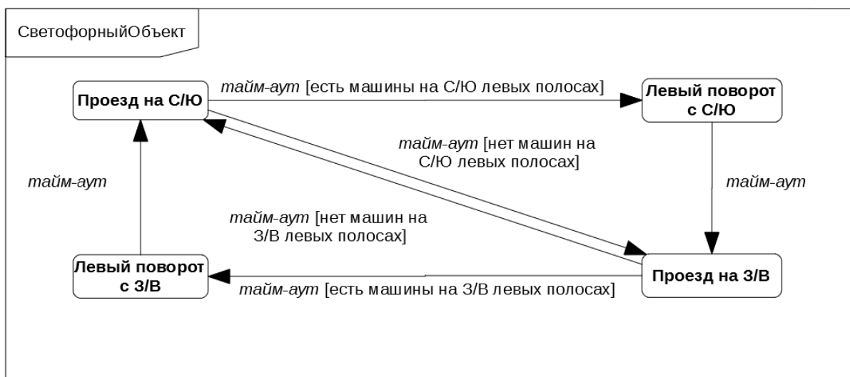
Рис. 4.14 – Переходы со сторожевými условиями
