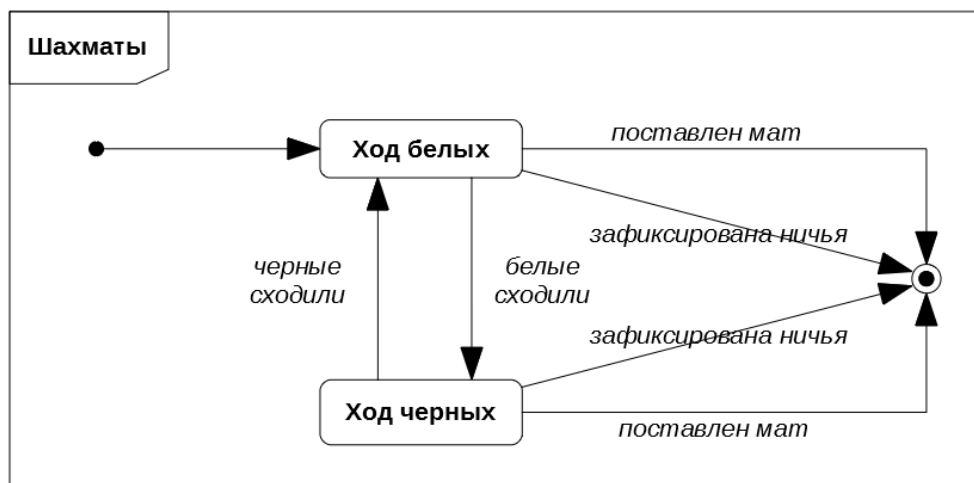
Рис. 4.15 – Диаграмма состояний игры в шахматы
