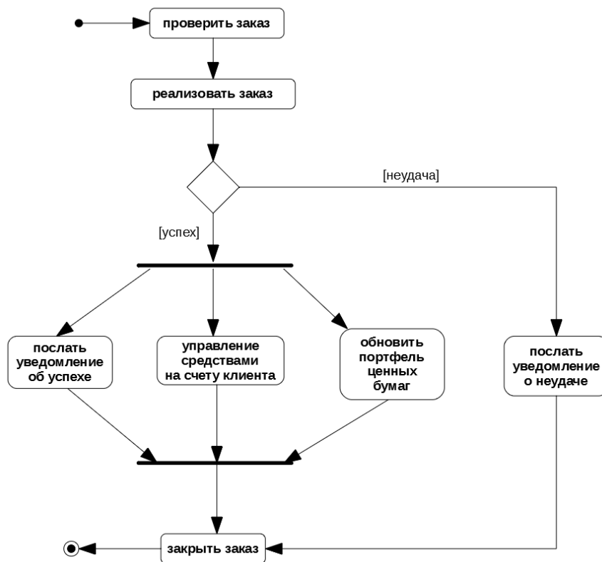
Рис. 4.20 – Диаграмма деятельности брокерской системы при обработке заказа
