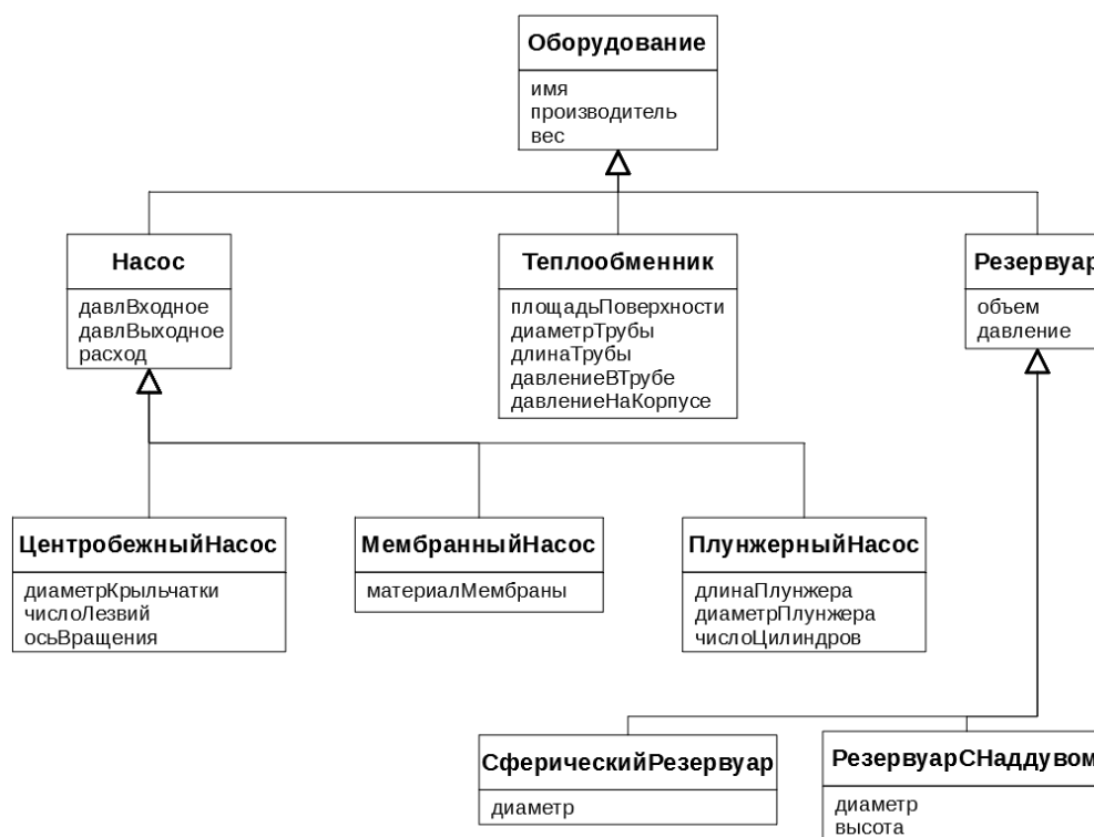
Рис. 4.10 – Многоуровневая иерархия наследования с экземплярами
