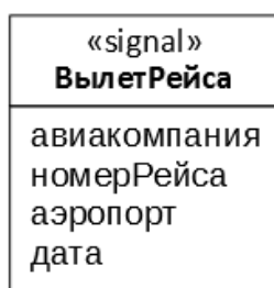
Рис. 4.11 – Класс сигналов и его атрибуты
