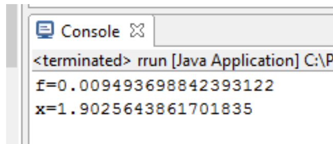
Рис. Г.18 – Результат программы
