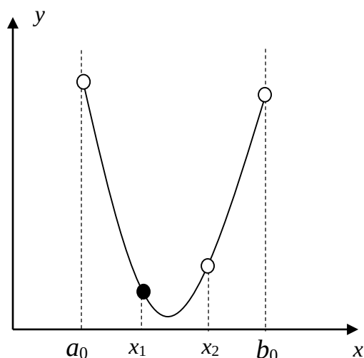
Рис. 1.2 – Метод равномерного поиска. Разбиение интервала на три подынтервала
