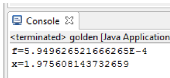
Рис. Г.20 – Результат работы программы
