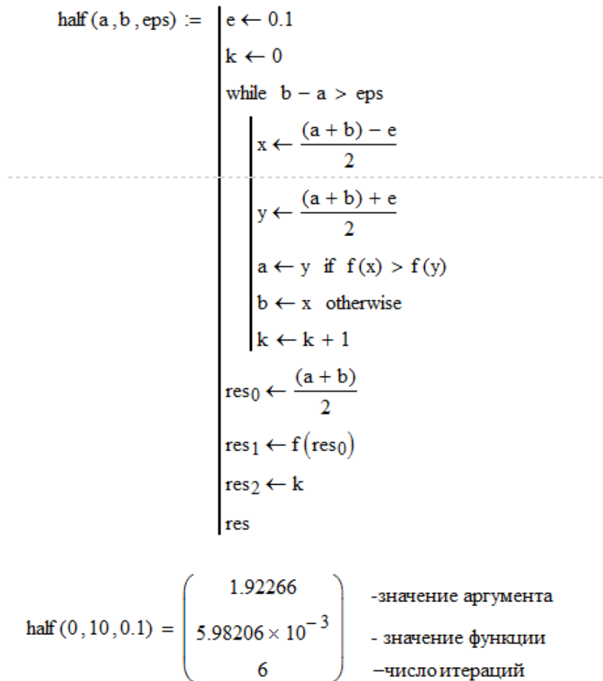
Рис. Г.14 – Определение числа итераций
