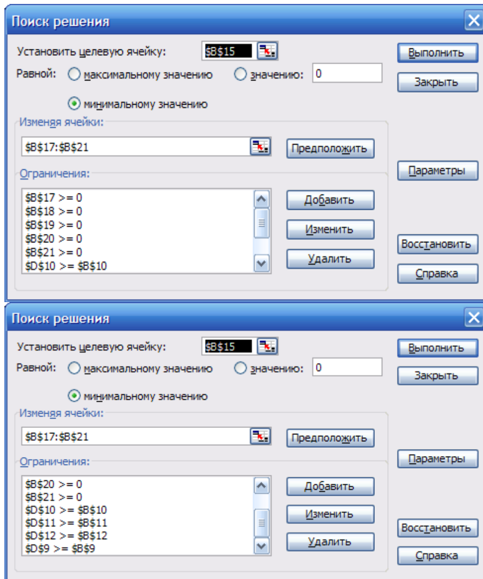
Рис. Г.38 – Надстройка «Поиск решения»
