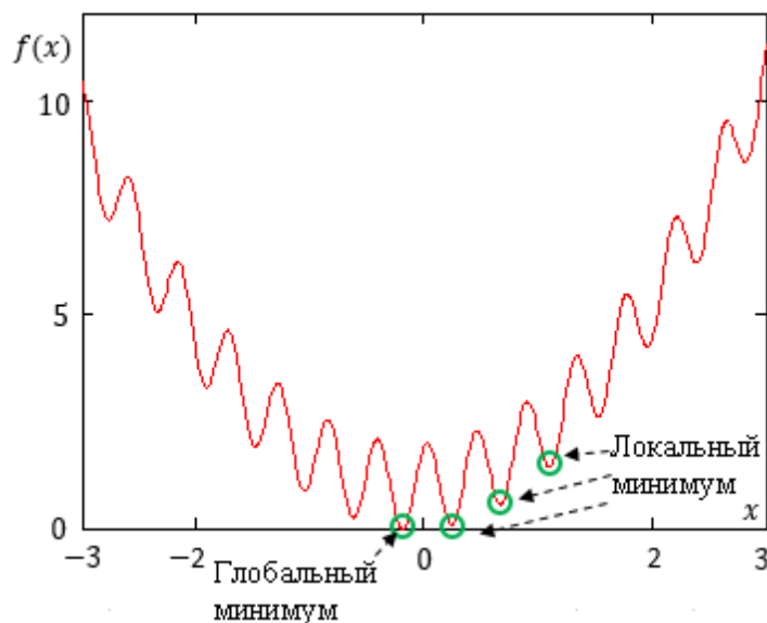
Рис. 1.1 – График функции f(x) = \cos(14,5x - 0,3) + x(x + 0,2) + 0,01
