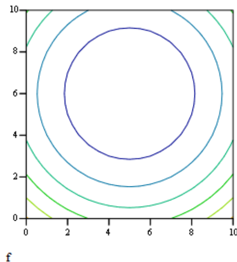
Рис. Г.28 – Контурный график
