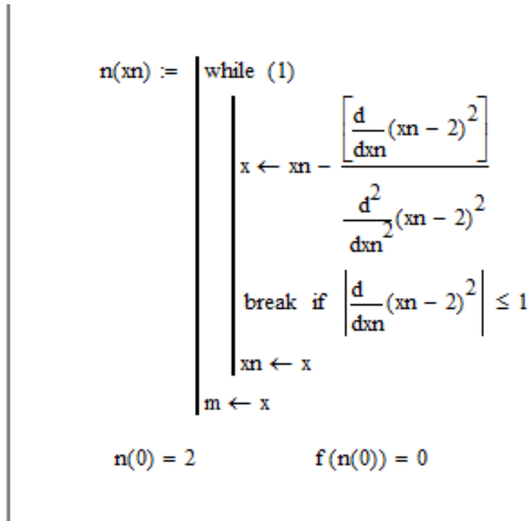
Рис. Г.13 – Решение задачи методом Ньютона
