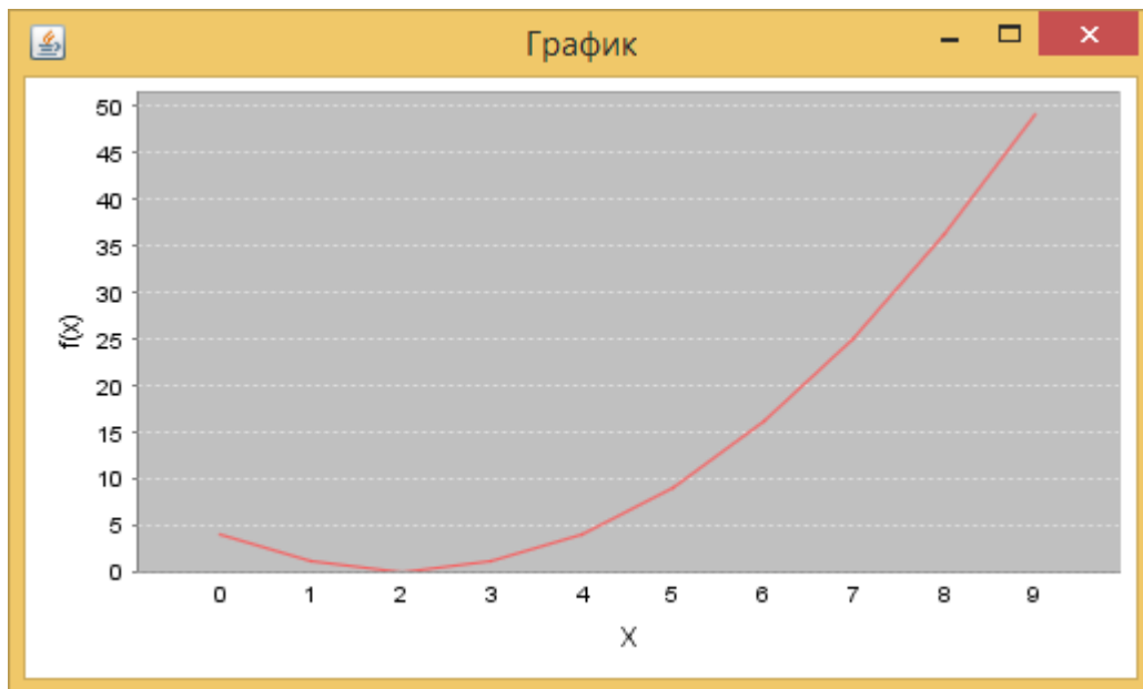
Рис. Г.15 – График функции f(x) = (x - 2)^2 на интервале [0;10]
