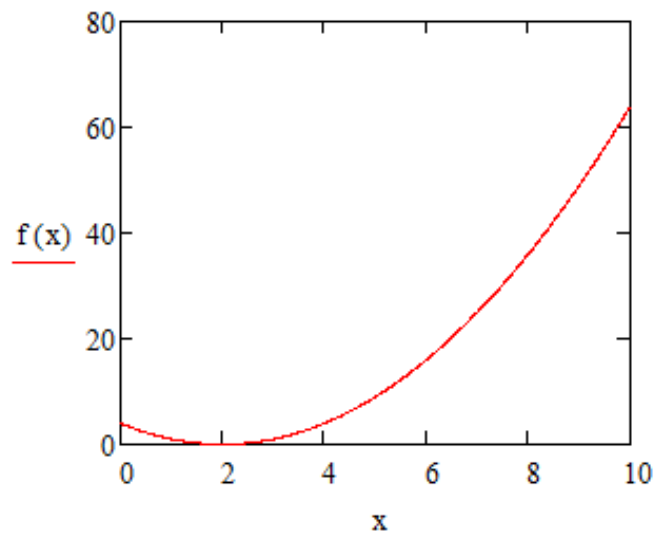
Рис. Г.9 – График функции f(x) = (x - 2)^2
