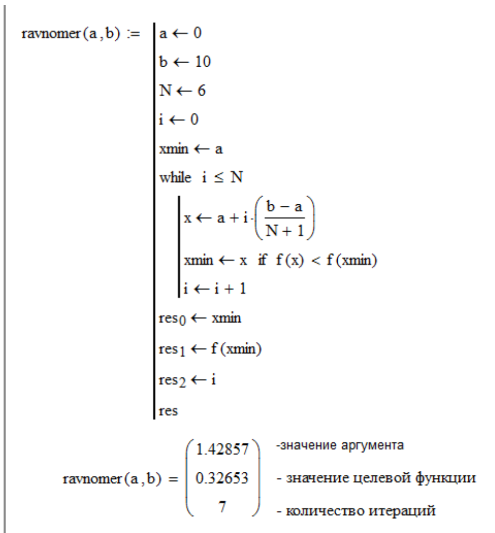
Рис. Г.11 – Реализация алгоритма равномерного поиска в MathCad
