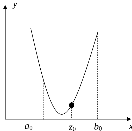
Рис. 1.7 – Производная в средней точке положительна, следовательно, правая граница будет смещена
