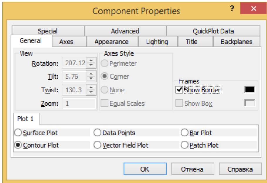
Рис. Г.27 – Построение контурного графика
