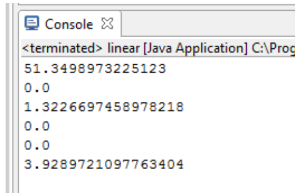
Рис. Г.47 – Результат работы программы
