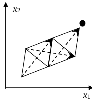
Рис. 2.3 – Движение симплекса
