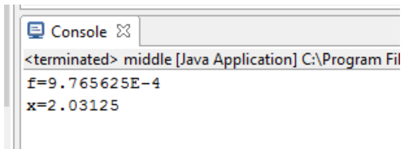
Рис. Г.22 – Результат работы программы
