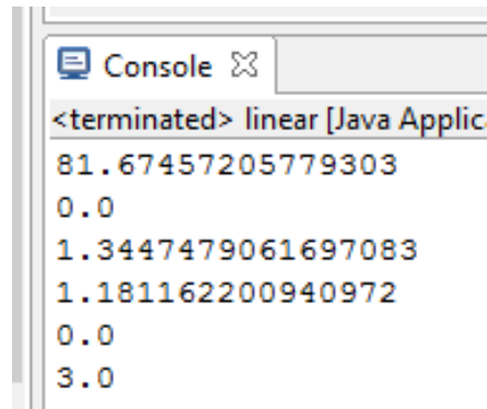
Рис. Г.49 – Результат работы программы
